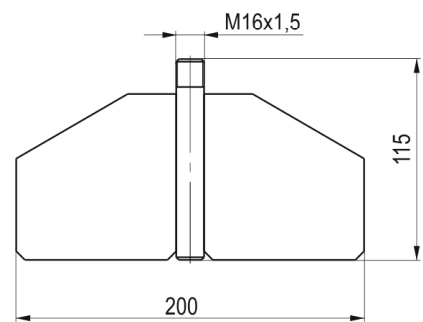
Удлинитель - Лопатка №2
