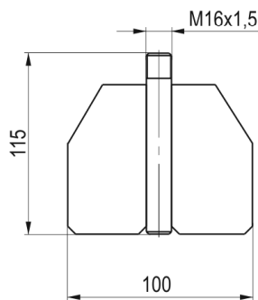
Удлинитель - Лопатка №1
